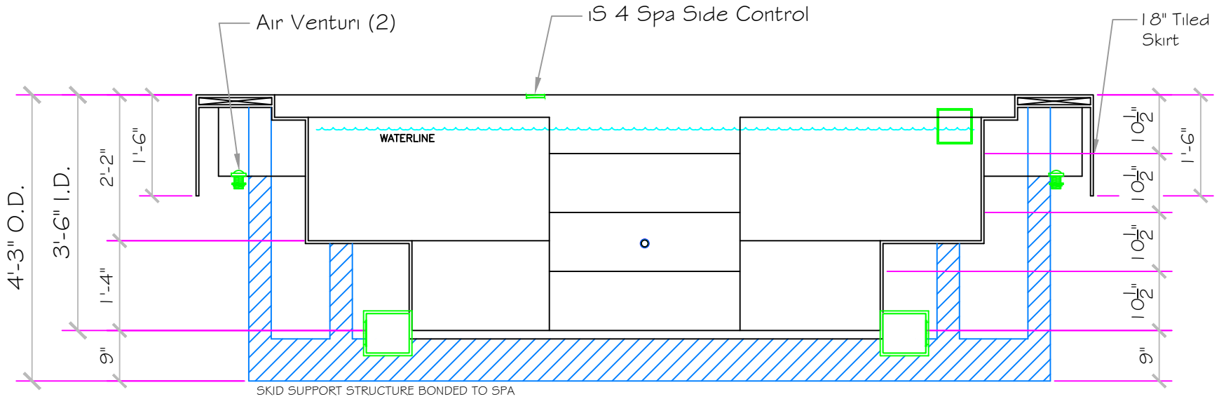
SECTION A-A
